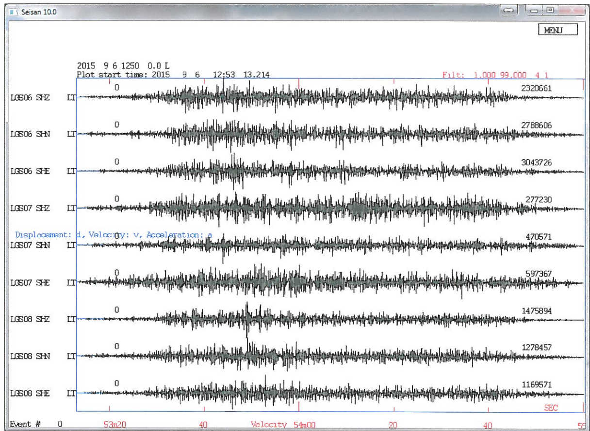
Attēls Nr. 18. Kravu dīzeļvilciena vibrāciju ieraksts Torņakalnā. Seismogramma rāda zemes virsmas svārstību ātruma laika vēsturi. Svārstību maksimālais ātrums ir attēlots seismogrammas labajā pusē, pie katras komponentes. Ātrumu mērvienības ir nanometri sekundē.
