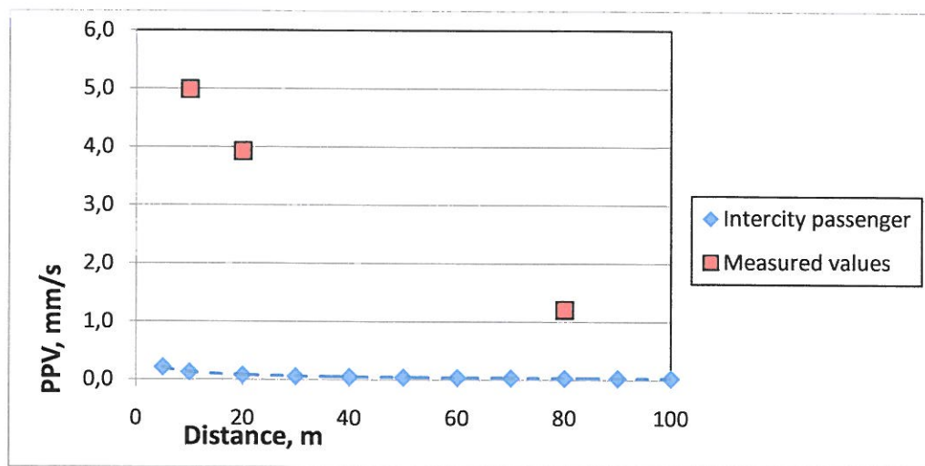
Attēls Nr. 20. Izmērītas PPV vērtības Sarkandaugavā (pasažieru elektrovilciens - sarkanie kvadrāti) un prognozētais vibrāciju līmenis pamatojoties uz Zviedru datiem (zilie rombi un pārtrauktā līnija).
