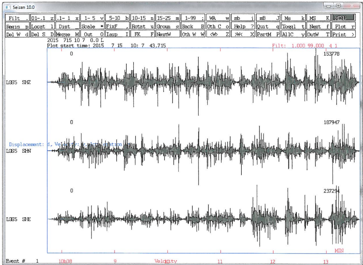
Attēls Nr. 4. Ierakstītas seismogrammas piemērs. Svārstības izmērītas uz ģipšakmens slāņa virsmas 50 metru attālumā no hidrauliskā āmura. Seismogrammas rāda zemes virsmas svārstību ātruma laika vēsturi. Katra mērījuma seismogramma ir uzrādīta ar trīs ortogonālajiem komponentiem: vertikālā (Z), ziemeļu-dienvidu (N) un austrumu-rietumu (E). Svārstību maksimālais ātrums ir attēlots seismogrammas labajā pusē, pie katras komponentes. Ātrumu mērvienības ir nanometri sekundē.
