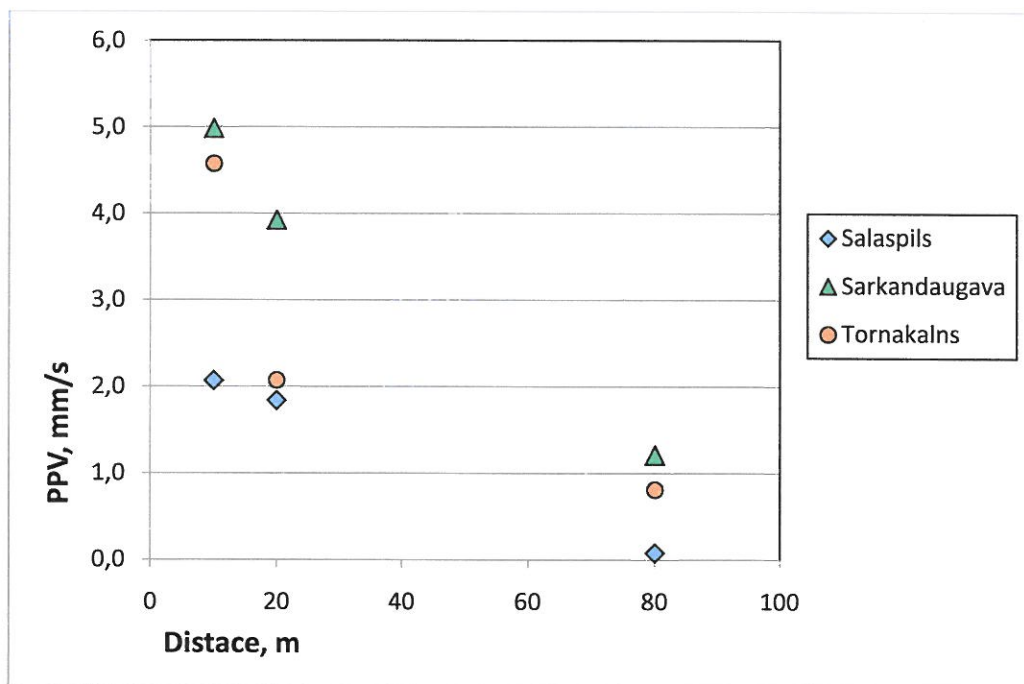
Attēls Nr. 19. Ierakstītas un uzņēmītas PPV vērtības trīs dažādās vietās – Salaspilī (pasažieru dīzeļvilciens), Sarkandaugavā (pasažieru elektrovilciens) un Torņakalnā (kravas dīzeļvilciens).
