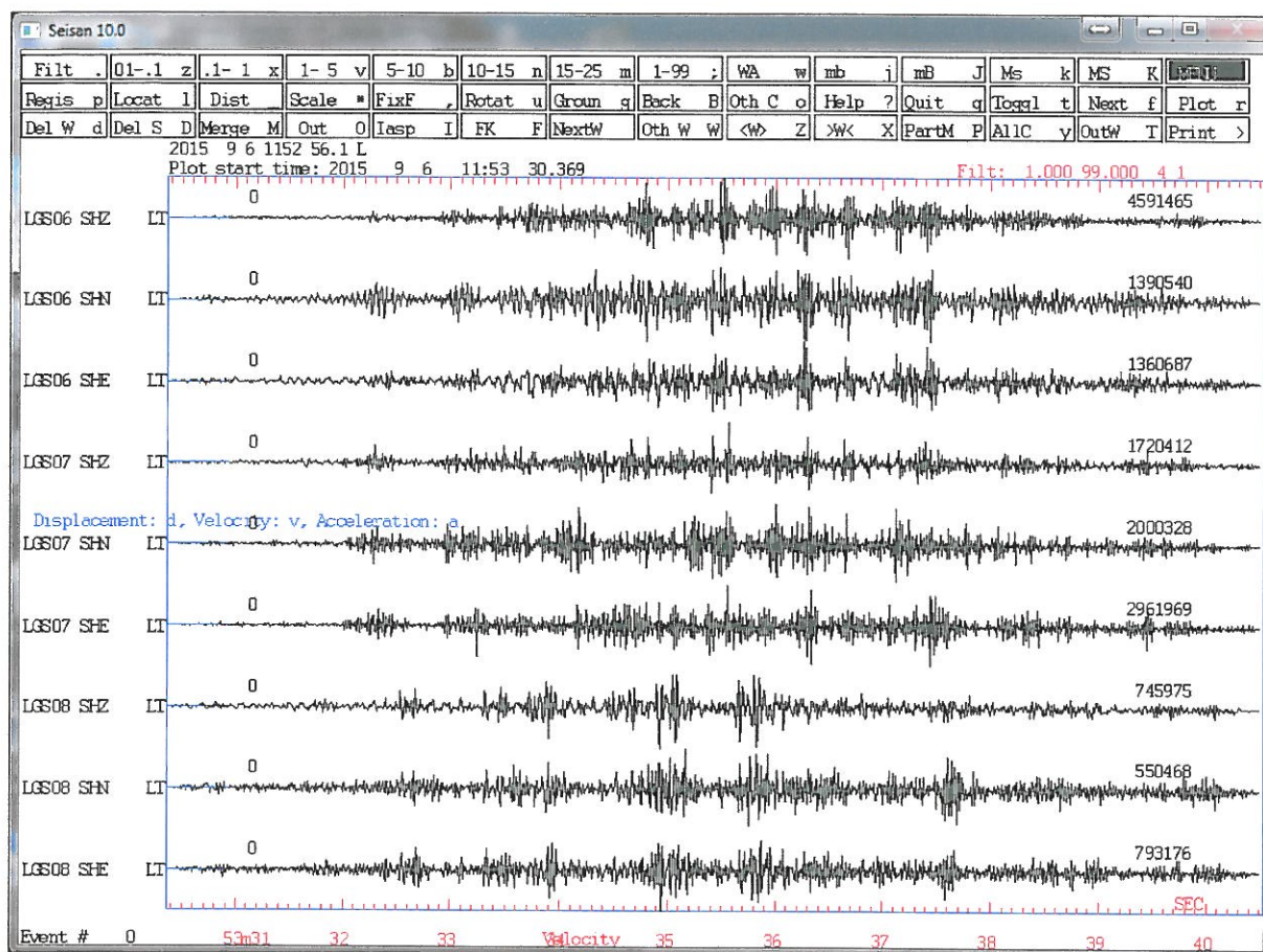
Attēls Nr. 17. Pasažieru elektrovilcienu vibrāciju ieraksts Sarkandaugavā. Seismogramma rāda zemes virsmas svārstību ātruma laika vēsturi. Svārstību maksimālais ātrums ir attēlots seismogrammas labajā pusē, pie katras komponentes. Ātrumu mērvienības ir nanometri sekundē.
