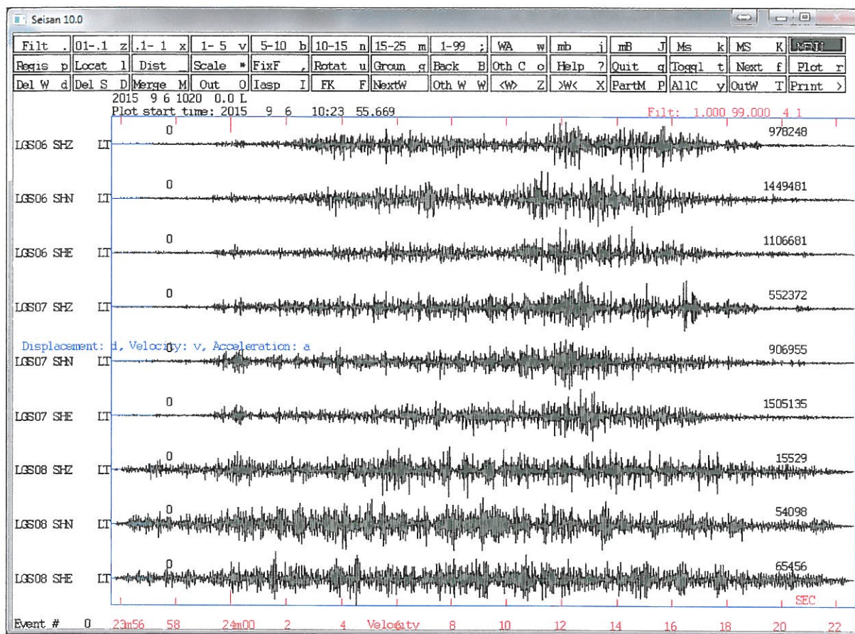
Attēls Nr. 16. Pasažieru dīzeļa vilciena vibrāciju ieraksts Salaspilī. Seismogramma rāda zemes virsmas svārstību ātruma laika vēsturi. Svārstību maksimālais ātrums ir attēlots seismogrammas labajā pusē, pie katras komponentes. Ātrumu mērvienības ir nanometri sekundē.
