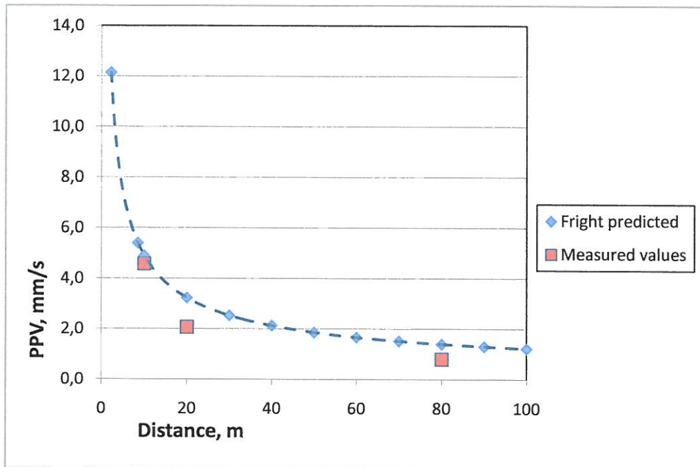
Attēls Nr. 23. Izmērītas PPV vērtības Torņakalnā (kravu dīzeļvilciens - sarkanie kvadrāti) un prognozētais vibrāciju līmenis pamatojoties uz Latvijā veiktiem mērījumiem (zilie rombi un pārtrauktā līnija).
