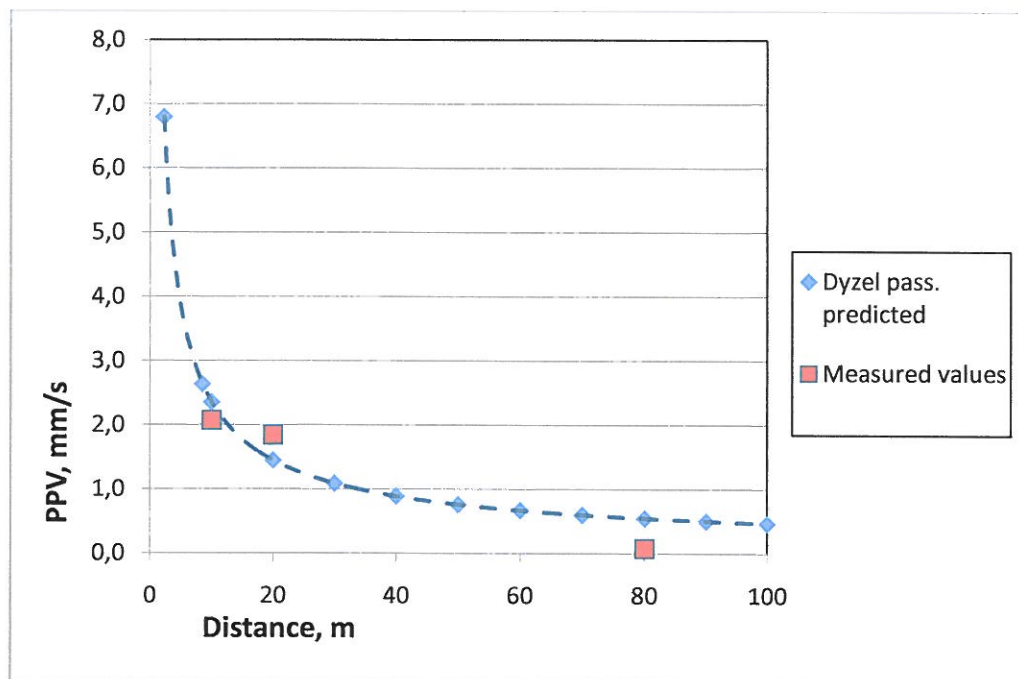
Attēls Nr. 21. Izmērītas PPV vērtības Salaspilī (pasažieru dīzeļvilciens - sarkanie kvadrāti) un prognozētais vibrāciju līmenis pamatojoties uz Latvijā veiktiem mērījumiem (zilie rombi un pārtrauktā līnija).
