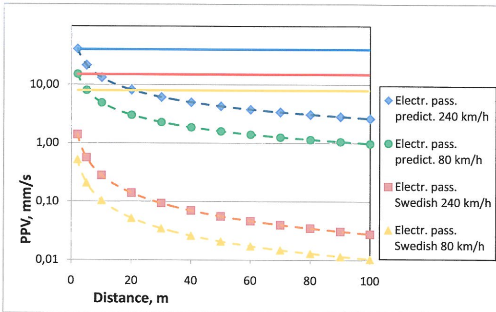
Attēls Nr. 24. Prognozētie vibrāciju līmeņi "Rail Baltica" pasažieru elektrorvilcieniem. Zilie rombi un zilā pārtrauktā līnija nozīme prognozētas vibrācijas pasažieru elektrorvilcieniem lauku rajonos (240 km/h), zaļie aplīši un zaļā pārtraukta līnija nozīme prognozētas vibrācijas pasažieru elektrorvilcieniem pilsētās (80 km/h), brūni kvadrāti un brūnā pārtraukta līnija nozīme vibrācijas pasažieru elektrorvilcieniem lauku rajonos Zviedrijā (240 km/h), dzeltenie trīsstūrīši un dzeltenā pārtraukta līnija nozīme vibrācijas pasažieru elektrorvilcieniem pilsētās Zviedrijā (80 km/h). Zilā nepārtraukta līnija norāda maksimāli atļauto vibrāciju līmeni pēc tabulas Nr. 1. pirmās rindas (industriālas ēkas). Sarkanā nepārtraukta līnija norāda maksimāli atļauto vibrāciju līmeni pēc tabulas Nr. 1. otras rindas (dzīvojamās ēkas un līdzīgas ēkas). Dzeltenā nepārtraukta līnija norāda maksimāli atļauto vibrāciju līmeni pēc tabulas Nr. 1. trešās rindas (struktūras, kas ir īpaši jutīgas pret vibrāciju).
