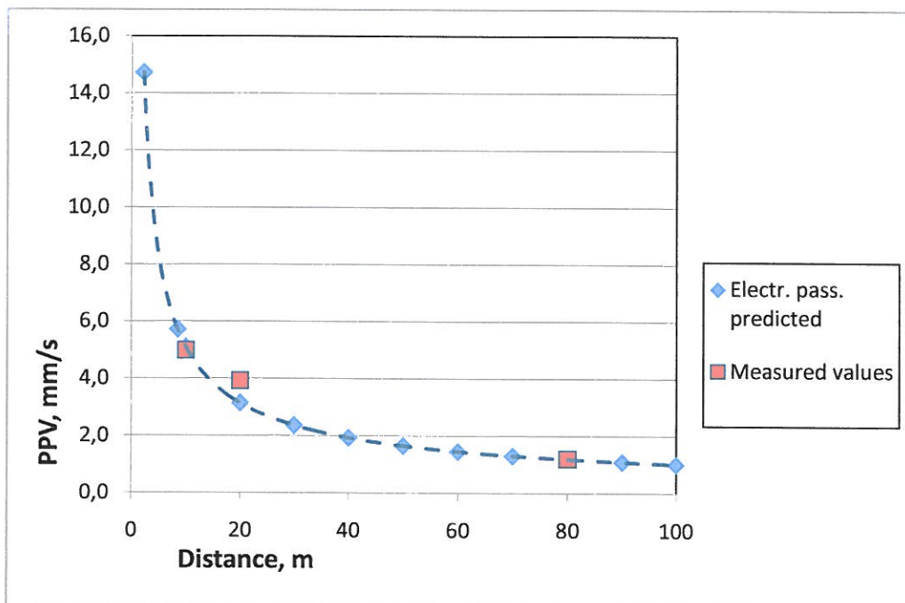
Attēls Nr. 22. Izmērītas PPV vērtības Salaspilī (pasažieru elektrovilciens - sarkanie kvadrāti) un prognozētais vibrāciju līmenis pamatojoties uz Latvijā veiktiem mērījumiem (zilie rombi un pārtrauktā līnija).
